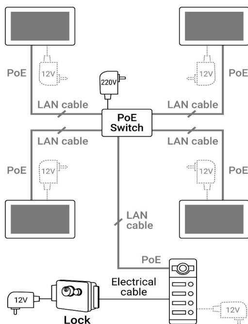
Схема монтажа
